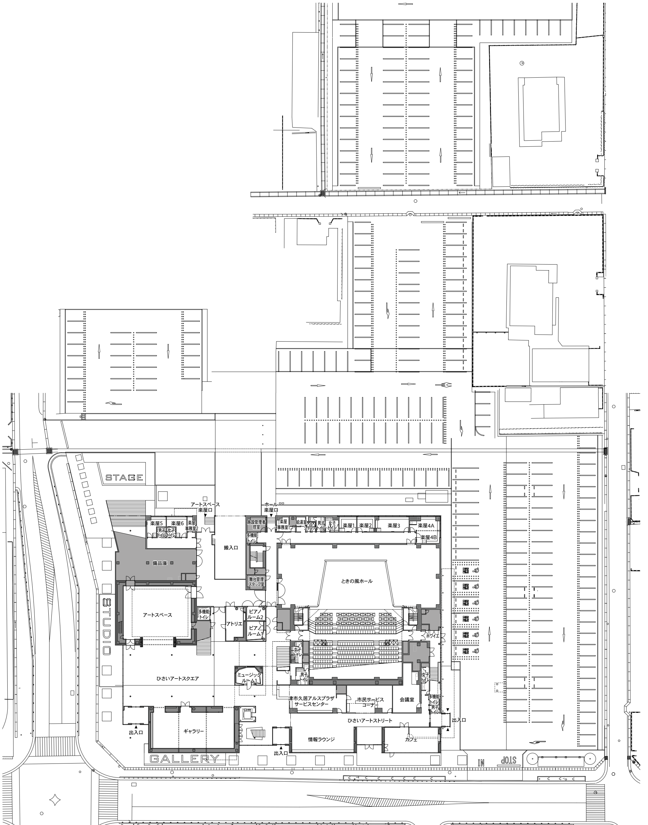
配置図 1:500 (A3印刷) 0 3 6 12m
