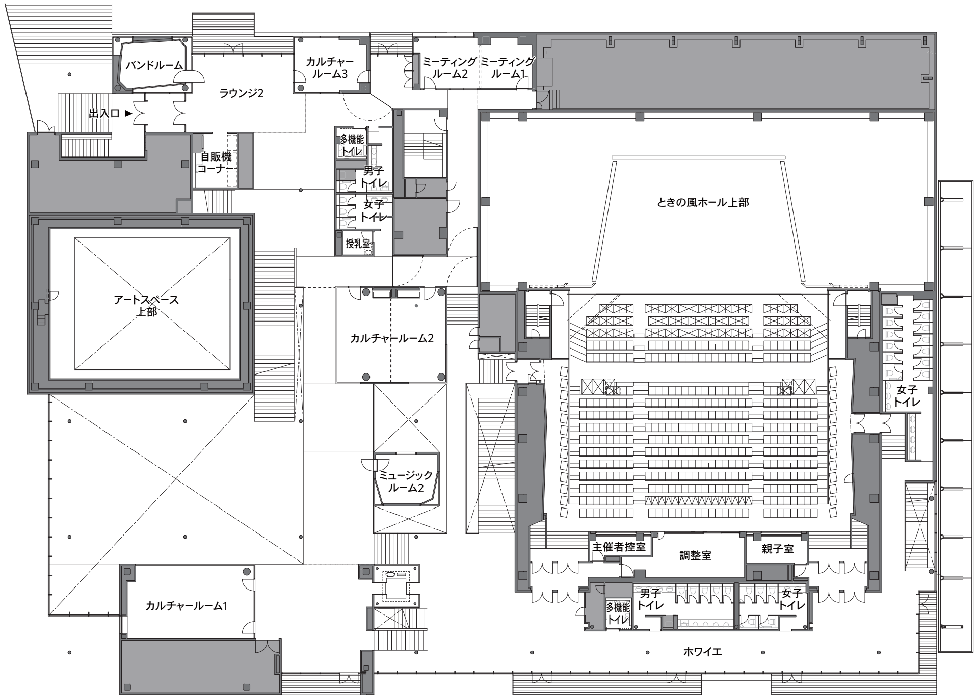
2F平面図 1:300 (A4印刷) 0 1 3 6m
